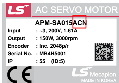
Incremental(증분형)
