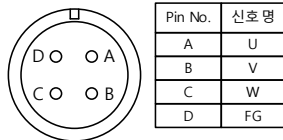
Plug : MS3102A22-22P
