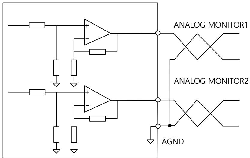
서보 드라이브
